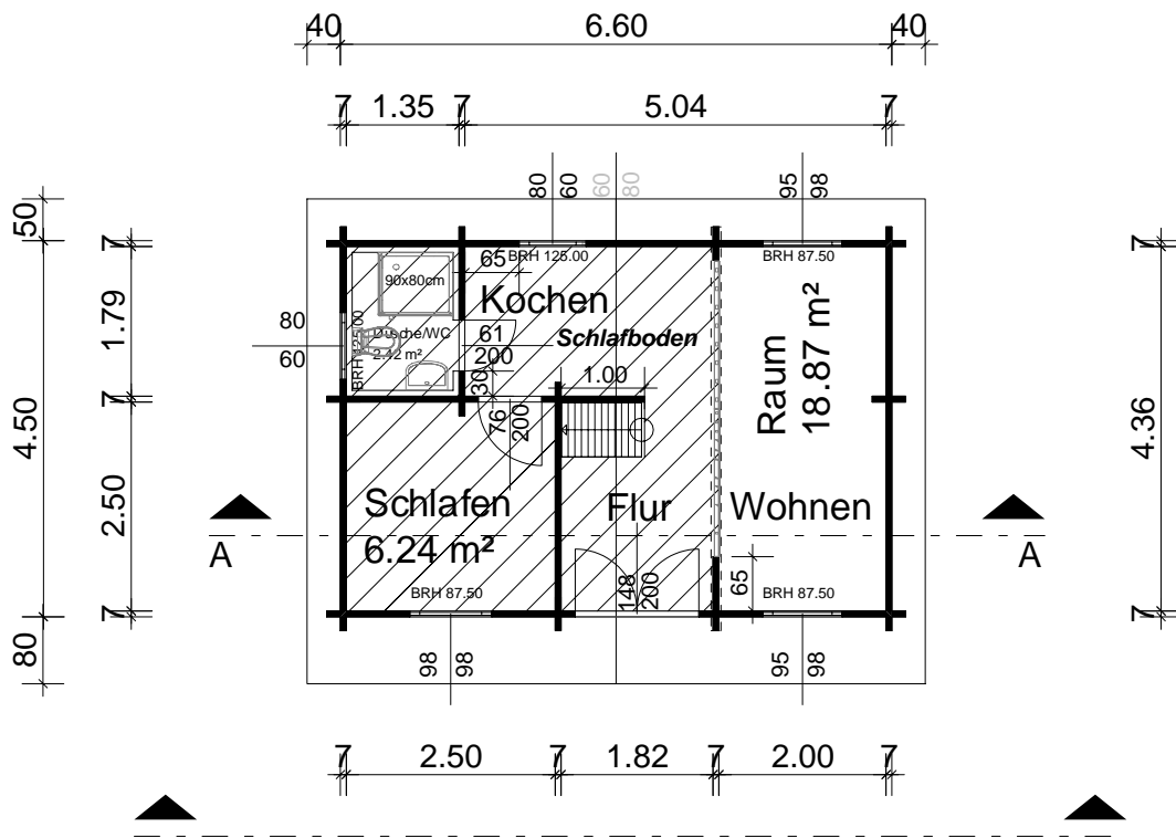
Schnitt A--A
